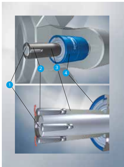
Principio del "movimento planetario": Il cono (1) è saldamente connesso al mandrino (4) e la punta (3) con i rulli rotanti inseriti (2) può girare liberamente.
