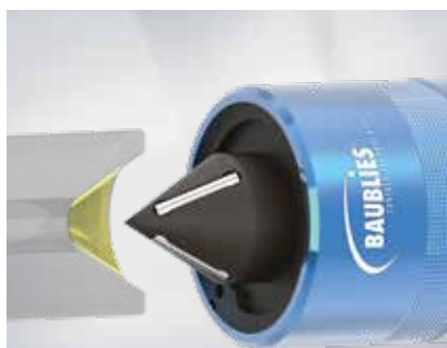
LUCIDATURA PER SUPERFICI CONICHE
